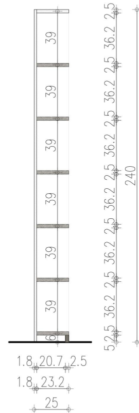
ПРЕСЕК 1-1
