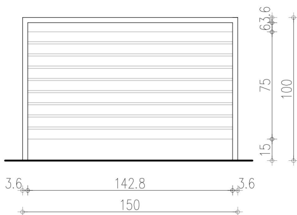
ИЗГЛЕД А
