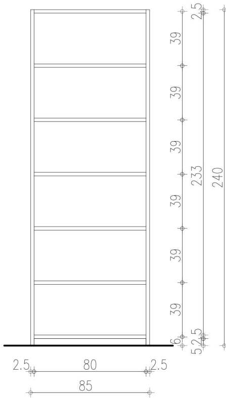
ИЗГЛЕД А
